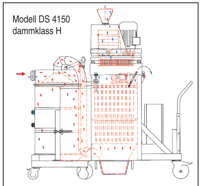
Föravskiljare på separat vagnstativ
